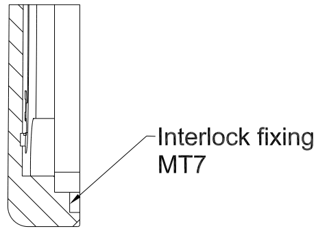
D-D ( 2 : 1 )
