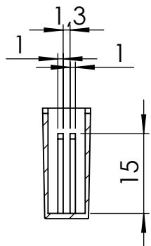
SEZIONE A-A
